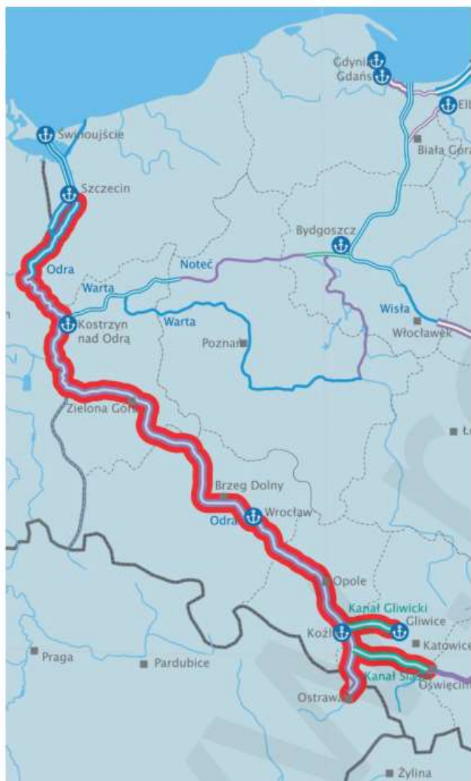
Rysunek 16. Odrzańska Droga Wodna E-30 – perspektywa 2030 r.
