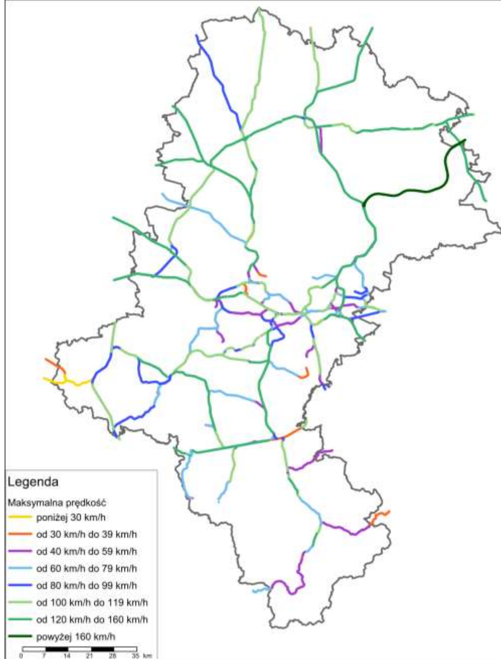
Rysunek 180. Maksymalne prędkości na liniach kolejowych w województwie śląskim.
