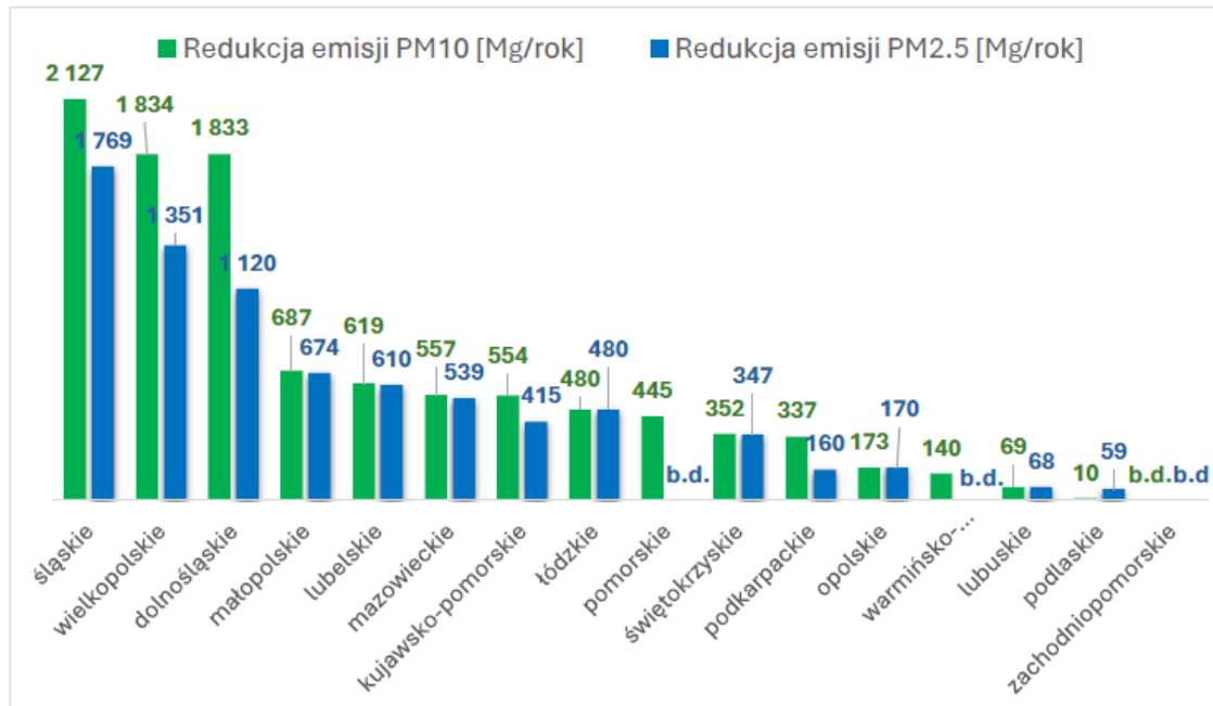
Wykres 6. Całkowita szacunkowa redukcja emisji dla pyłu PM10 i PM2.5 w 2024 r.
