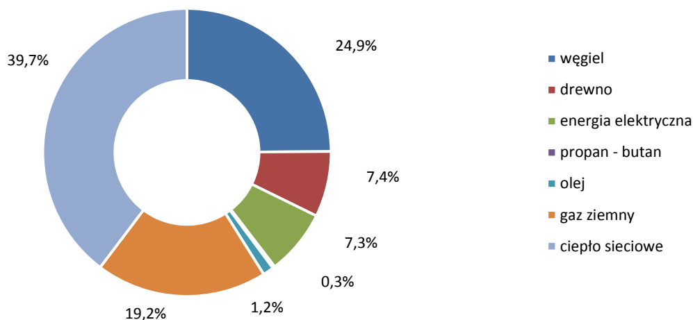
Rysunek 3-4 Struktura zużycia paliw i energii elektrycznej na cele grzewcze – ogrzewanie pomieszczeń
