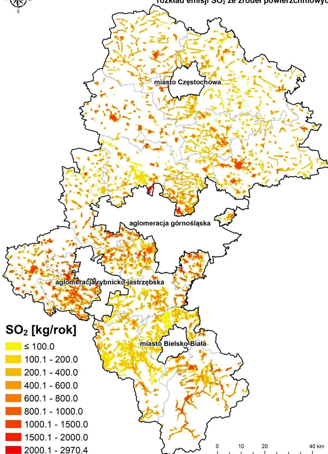
Rysunek 39. Lokalizacja i wielkość emisji dwutlenku siarki ze źródeł powierzchniowych w strefie śląskiej w roku bazowym 2015 133
