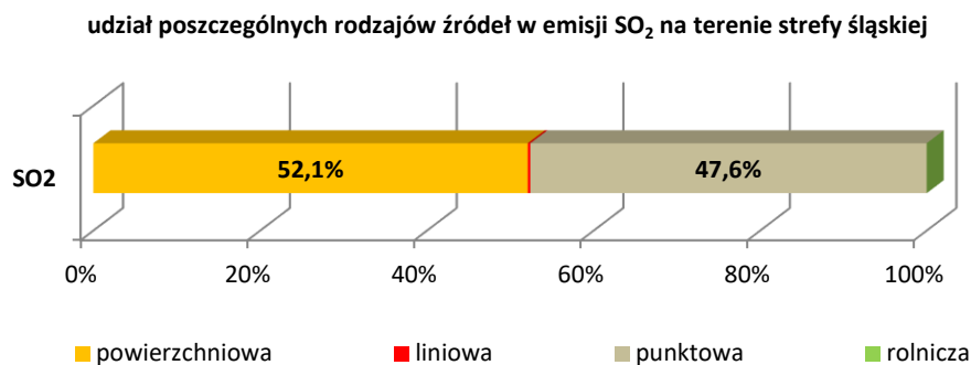
Rysunek 13. Udział poszczególnych rodzajów źródeł w emisji dwutlenku siarki na terenie strefy śląskiej w roku bazowym 2017
